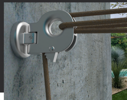
Réf : 280 56 587 Poulie monobloc 6:1 sur embase simple
